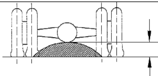
Рисунок 5. Дорожный просвет под одной осью
