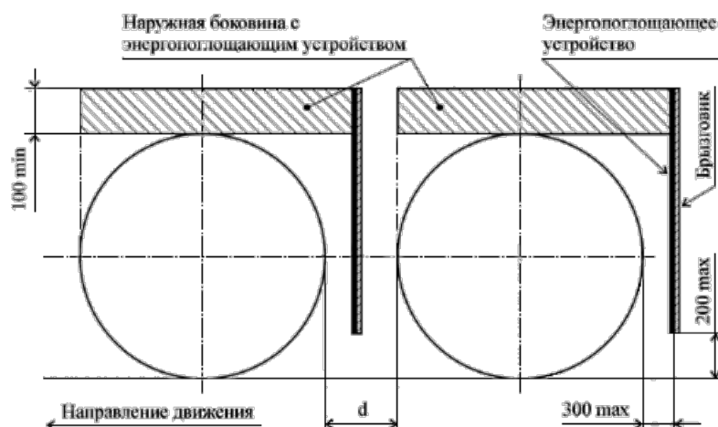
Рисунок 9.4 - Схема системы защиты от разбрызгивания с энергопоглощающими устройствами для осей с неуправляемыми и самоуставляющимися колесами
